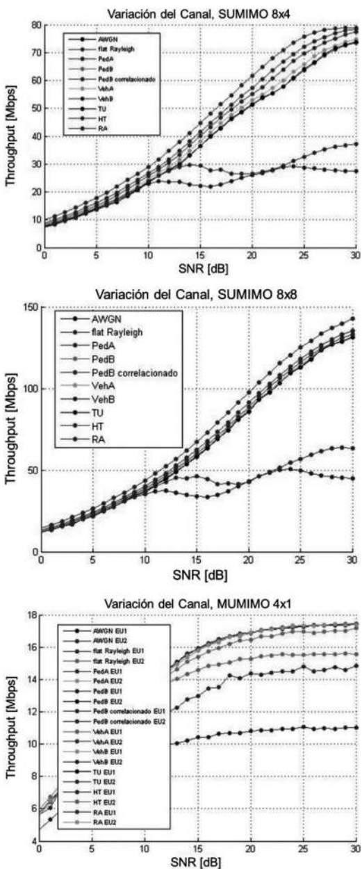
Figura 8. Variación del Tipo de Canal en LTE. Throughput.
