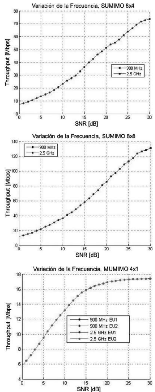
Figura 4. Variación de la frecuencia en LTE-Advanced. Throughput.
