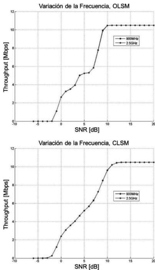
Figura 3. Variación de la frecuencia en LTE. Throughput.
