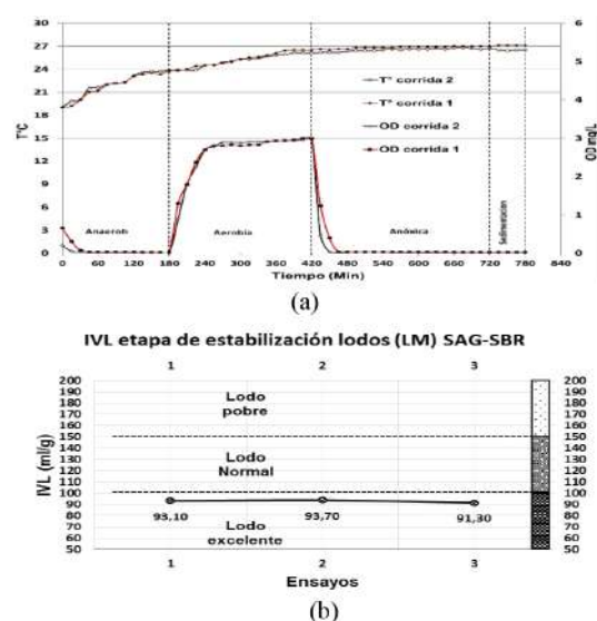
Figura 4. (a) Variación de T y OD; (b) IVL etapa de estabilización lodos (LM) SAG-SBR.
