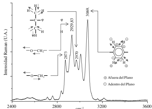
Figura 16. Representación de los modos normales de vibración para la resina DGEBA en el intervalo de 2400-3600 \text{cm}^{-1} .
