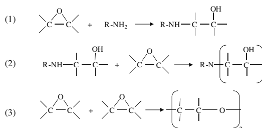
Figura 3. Mecanismo de reacción simplificado entre aminas y grupos epóxicos.
