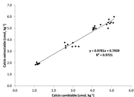
Figura 4. Correlación entre los contenidos de calcio extractable (Mehlich-3) y calcio cambiante (KCl 1N) de un suelo ácido enmendado con cáscara de huevo molida a los 135 días de incubación.
