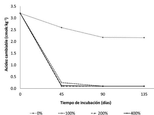
Figura 1. Efectos de la aplicación de cáscara de huevo molida sin tamizar (dosis equivalentes a 0, 100, 200 y 400% de la acidez cambiante) sobre la acidez cambiante de un suelo ácido durante un periodo de incubación de 135 días.
