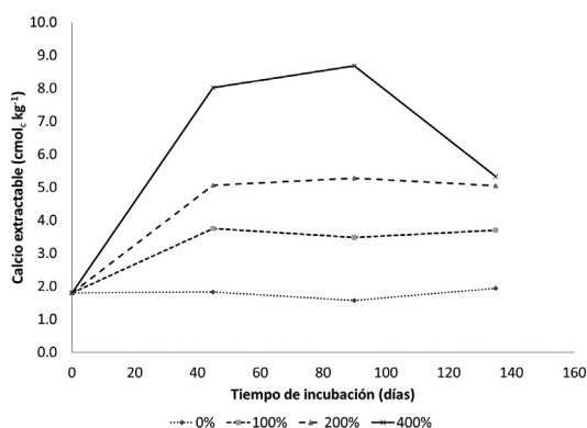
Figura 3. Efectos de la aplicación de cáscara de huevo molida sin tamizar (dosis equivalentes a 0, 100, 200 y 400% de la acidez cambiante) sobre el contenido de calcio extractable (Mehlich-3) de un suelo ácido durante un periodo de incubación de 135 días.
